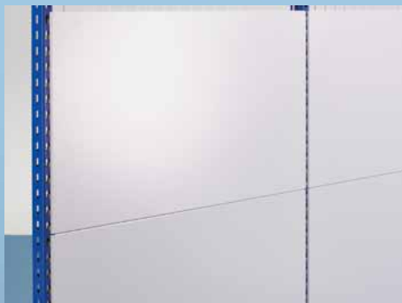
Vollblechwand als Sichtschutz oder Infowand zu nutzen. Systembreite 625, 1000 und 1250 mm, Höhe 380 und 590 mm. Auch vor Gitterelement einhängbar.
