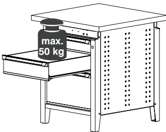
Schubladen mit Einfachauszug E 80 80% Auszug, 80 kg belastbar
